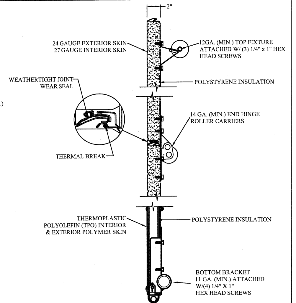
SECTION A-A (SIDE VIEW) N.T.S.
