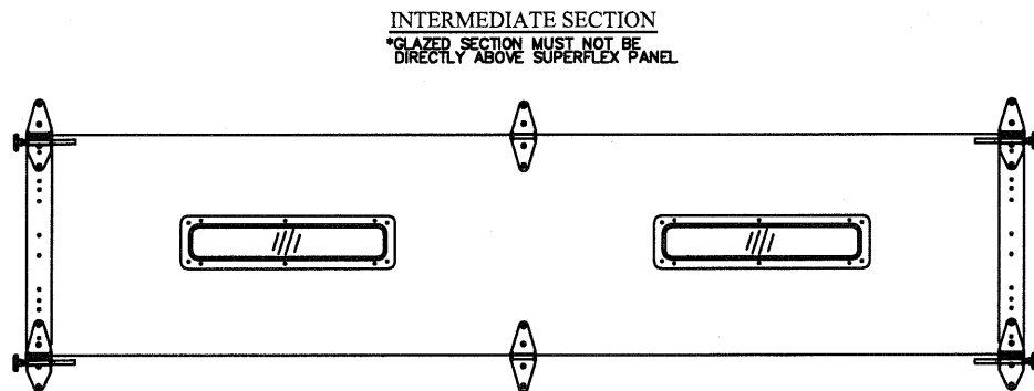
OPTIONAL GLAZED SECTION W/ 24" X 6" WINDOWS N.T.S.
