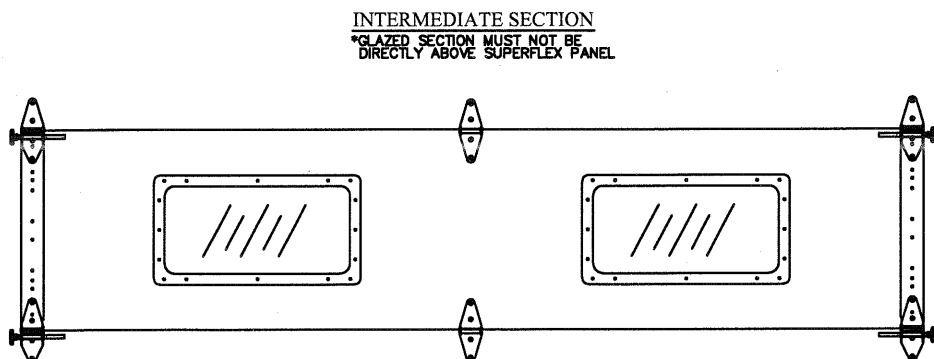
OPTIONAL GLAZED SECTION W/ 24" X 12" WINDOWS N.T.S.
