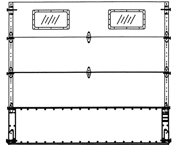
OPTIONAL SINGLE SUPERFLEX SECTION N.T.S.
