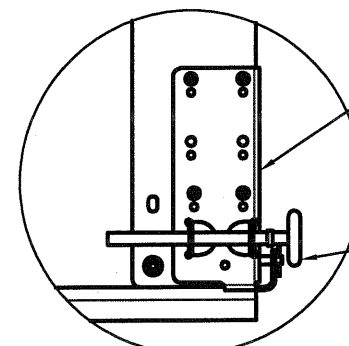
TYPICAL BOTTOM BRACKET N.T.S.
